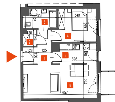
Rzut lokalu
