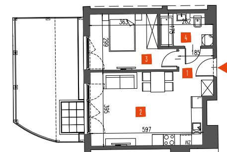
Rzut lokalu
